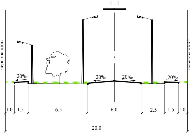
ПОПЕРЕЧНІ ПРОФІЛІ М 1:200
